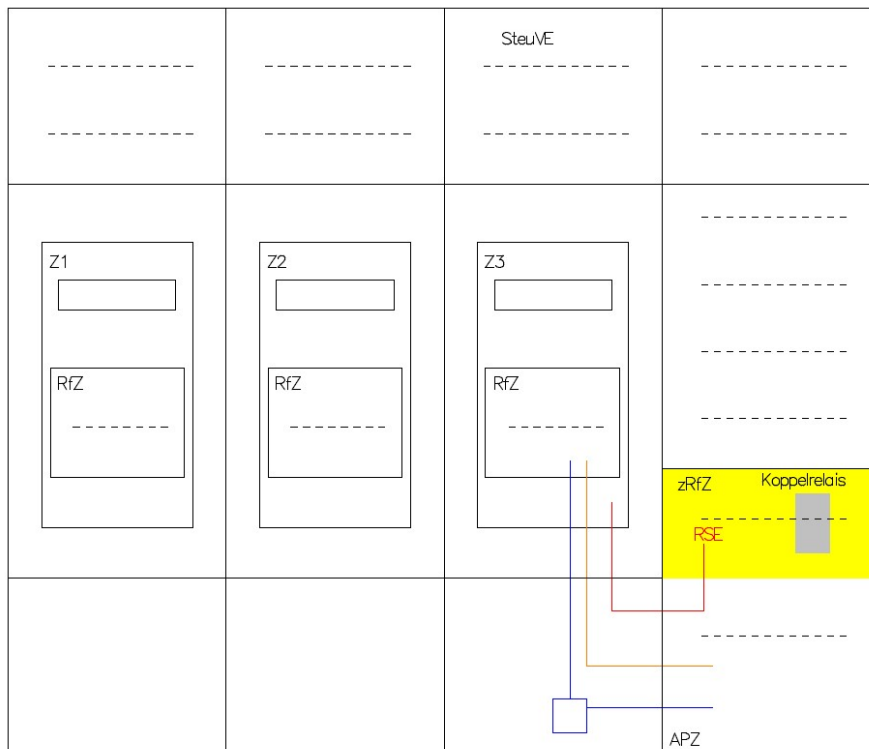
Abbildung 6: Mind. drei Zähler in einer Kundenanlage
