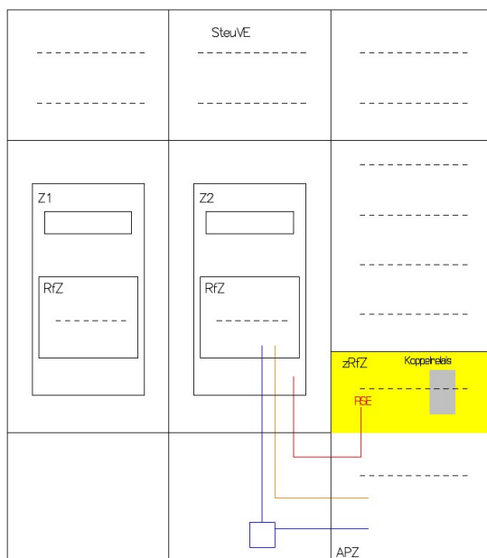
Abbildung 4: 2 Zählerplätze in einer Kundenanlage in Dreipunkt
