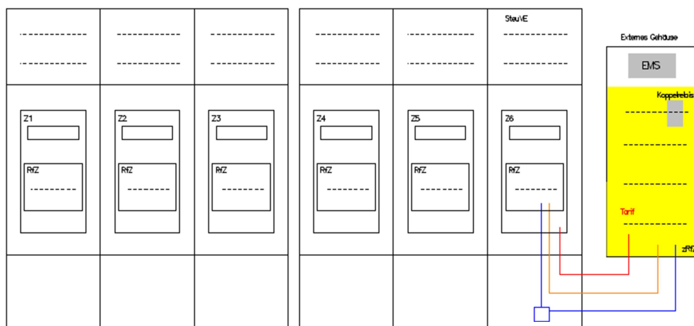
Abbildung 10: Bestandszählerplätze ohne zusätzlichen Zählerplatz bzw. Steuergerätefeld
