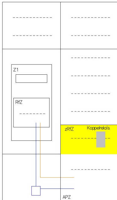
Abbildung 3: 1 Zähler in Kundenanlage in Dreipunkt
