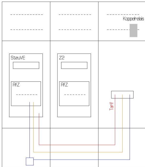
Abbildung 9: Bestandszählerplatz mit einem Steuergerätefeld
