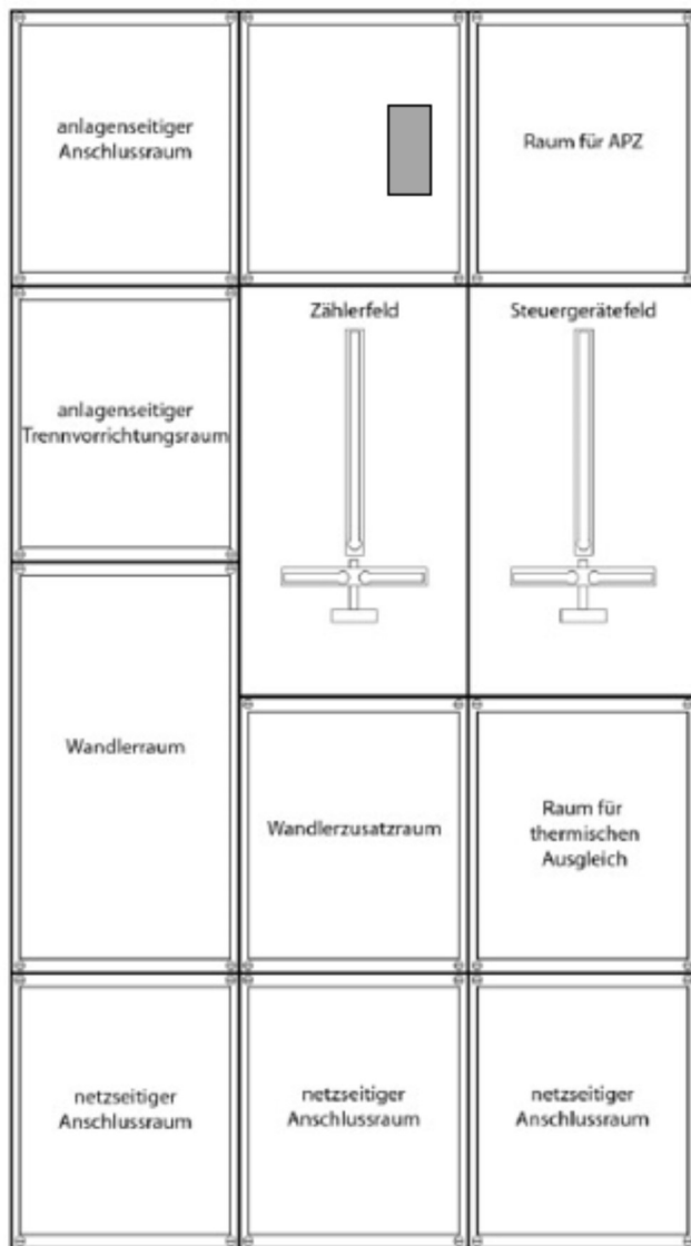
Abbildung 7: Bsp. Wandlerraummessung 200 A in Neuanlagen
