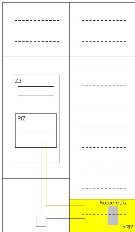
Abbildung 8: Bestandszählerplatz mit einem 1-feldrigen Zählerfeld
